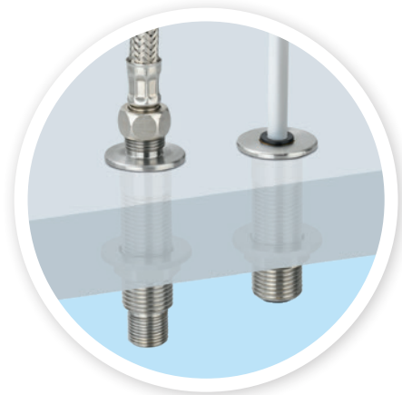
PIANI DI LAVORO PERFORATI professionali e pratici
